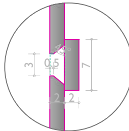
Detalj E - ručka
