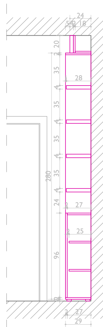
PRESEK 1-1
