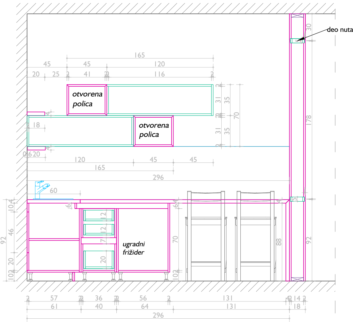
IZGLED B
