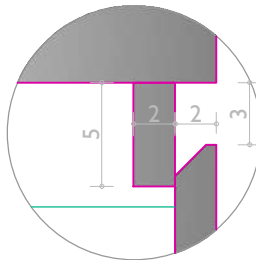
Detalj D - ručka
