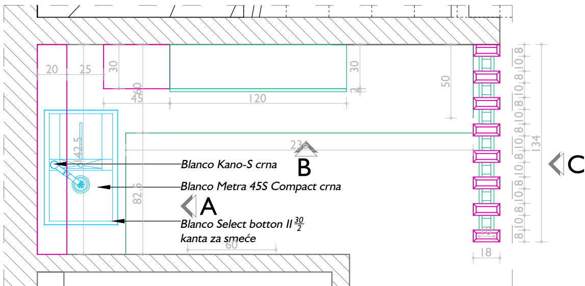
OSNOVA GORNJIH ELEMENATA
