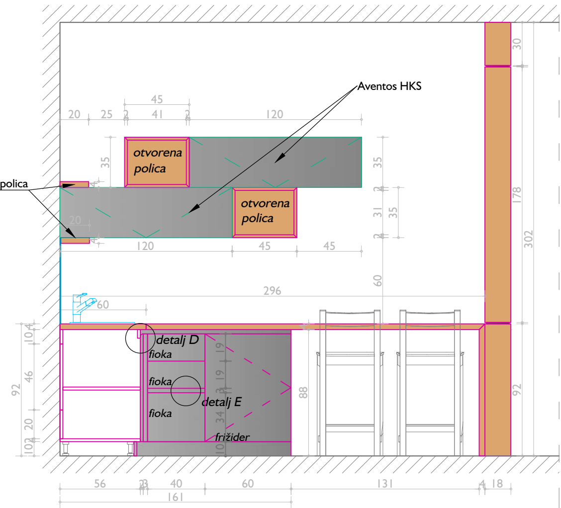
IZGLED B
