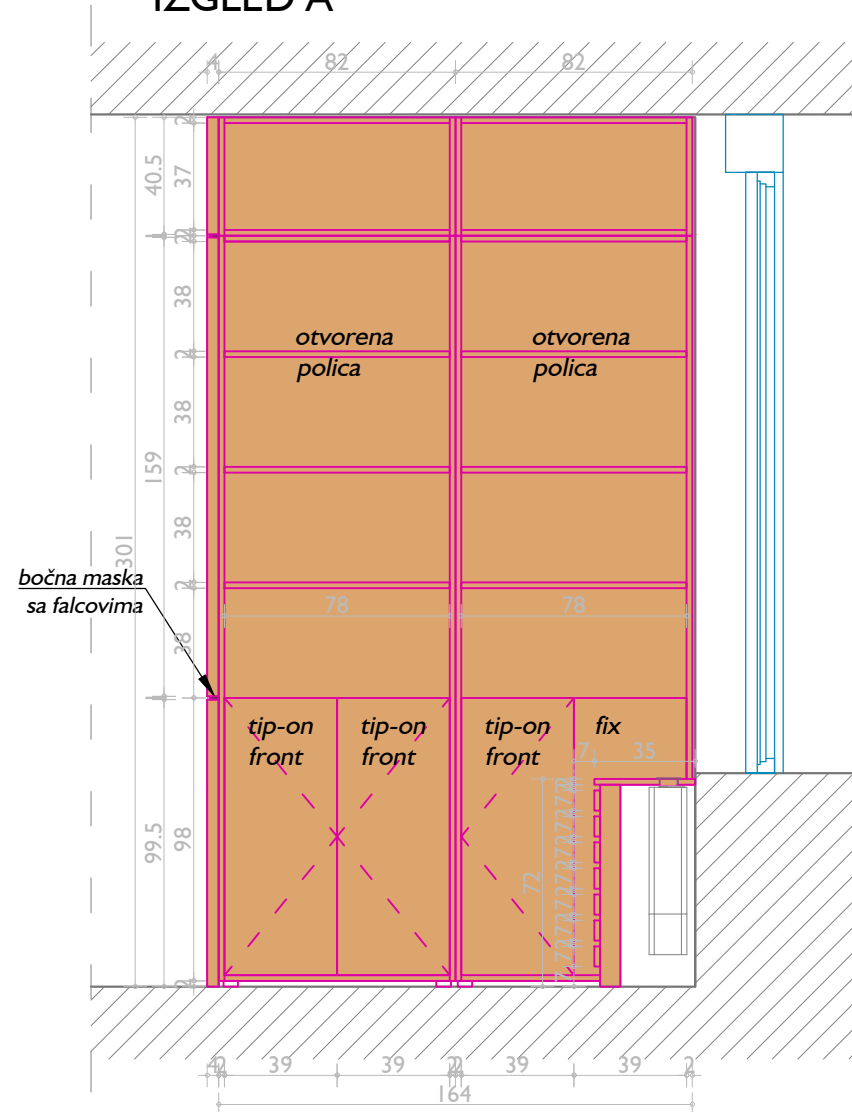
IZGLED A
