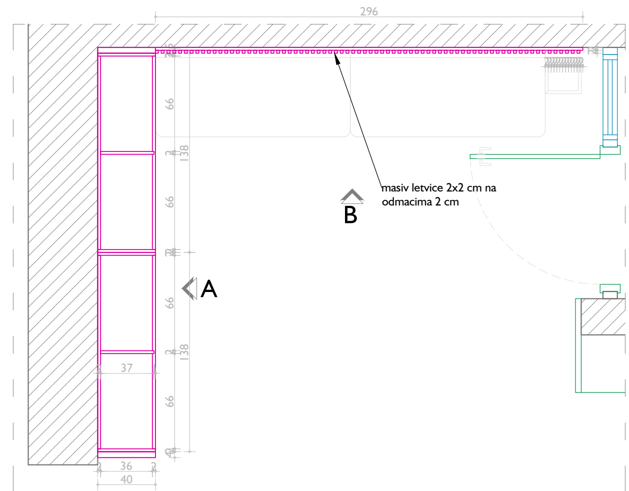
OSNOVA b-b
