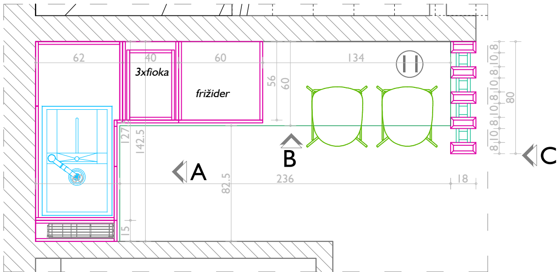
OSNOVA DONJIH ELEMENATA
