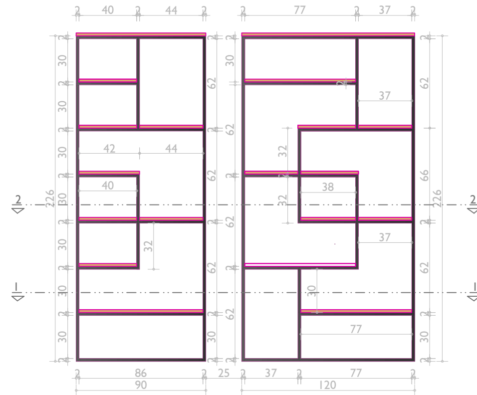
IZGLED A
