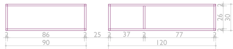
OSNOVA 1-1
