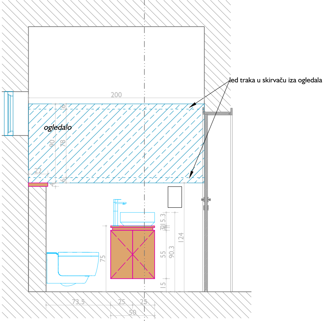
IZGLED A
