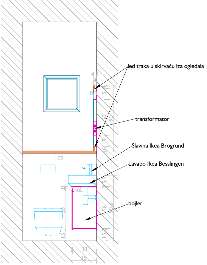
PRESEK I-I
