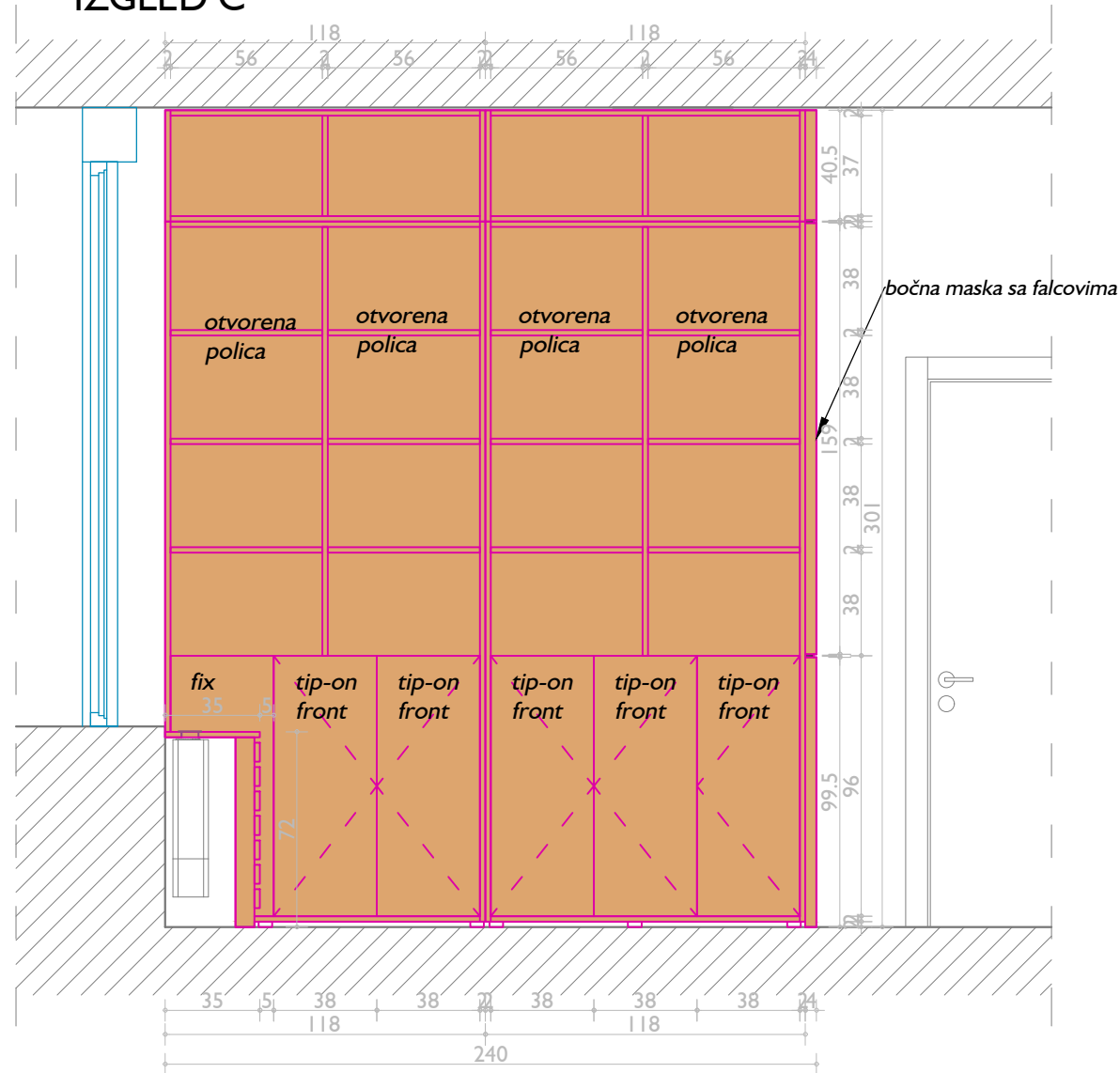
IZGLED C
